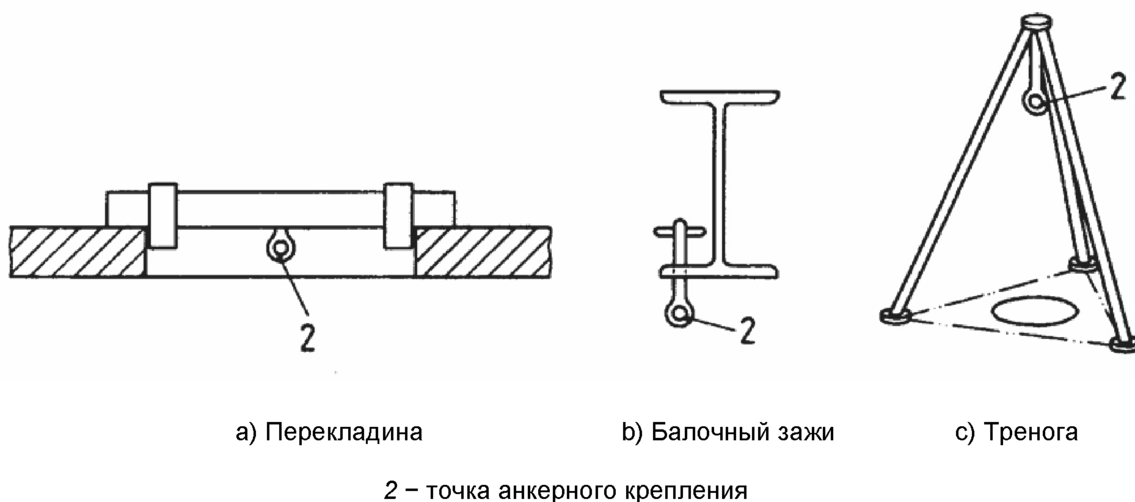
Рисунок 3 – Класс В. Примеры переносных временных анкерных устройств
